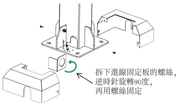
圖 3.2.2.2 (3) 立柱背部穿線
