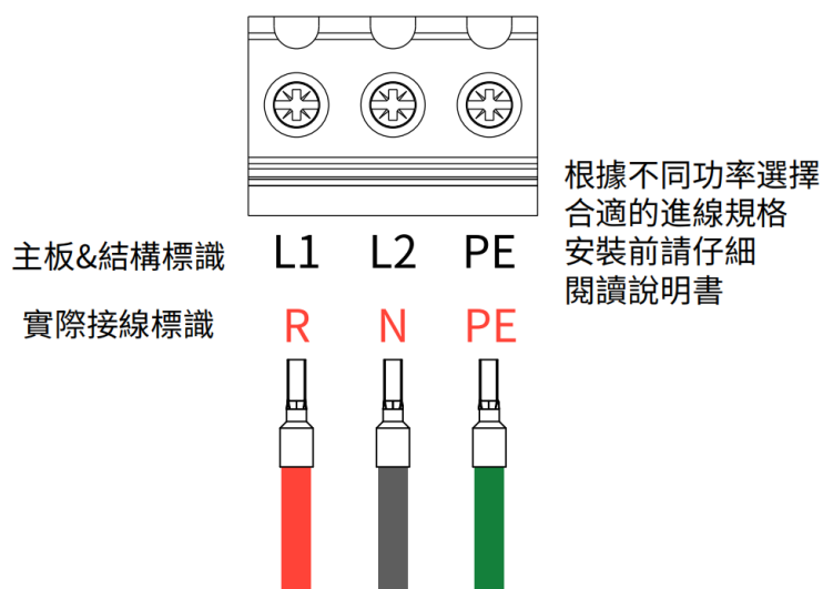
3.2.2.1 (8b) 接線
