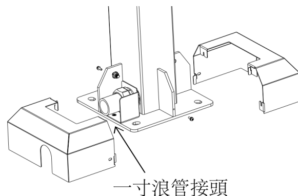
圖 3.2.2.2 (4) 立柱背部穿線
