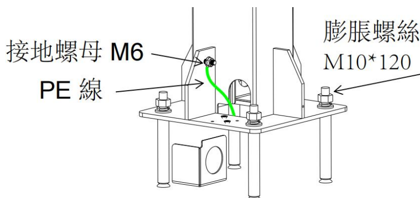
圖 3.2.2.2 (5) 立柱接地
