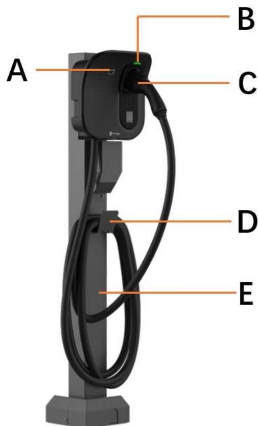
圖 2.2.2 電動車專用交流充電樁立柱式
