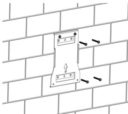
圖 3.2.2.1 (4) 固定壁掛件
